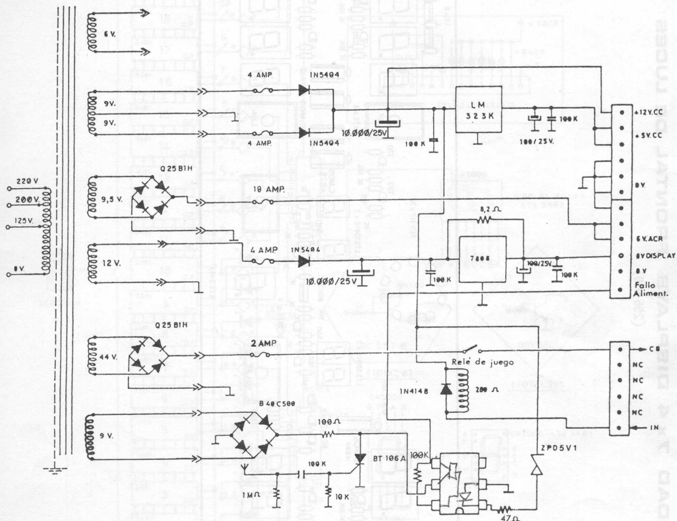
CIRCUITO ANTICHISPA
